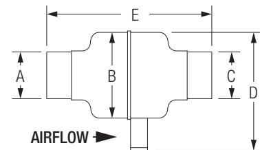
SF200
