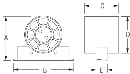
SF125 / SF100
